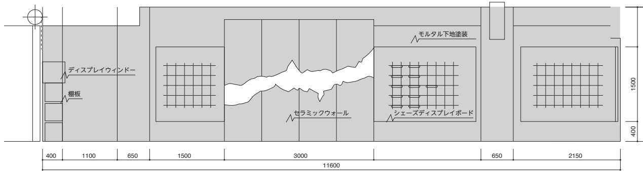
A 展開図
