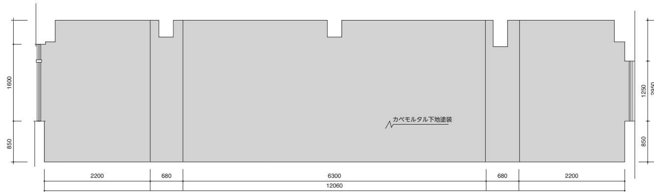
A 展開図
