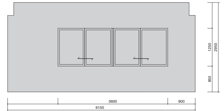
B 展開図
