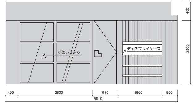
D 展開図
