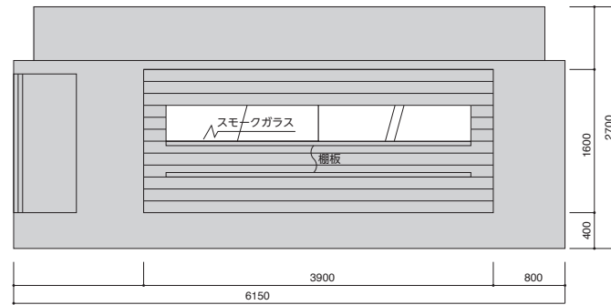
B 展開図
