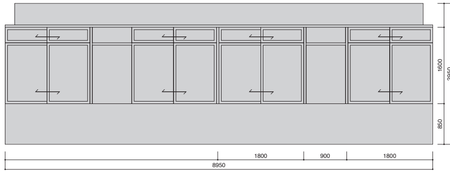
D 展開図
